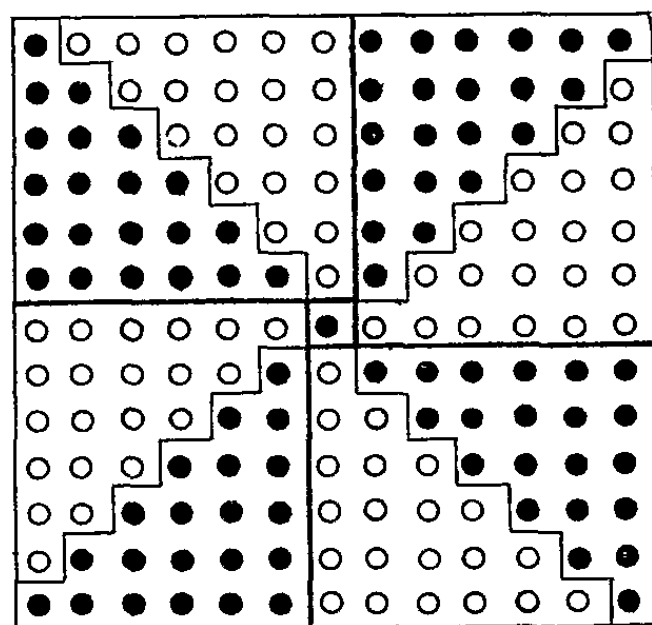
Un théorème de Diophante.
