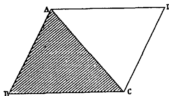
L'aire du triangle.
