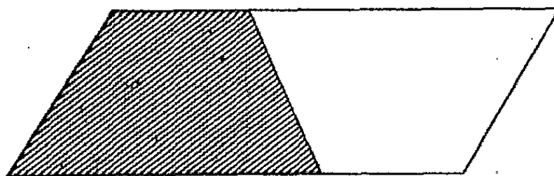
L'aire du trapèze.
